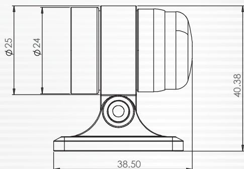
外觀尺寸圖 單位：mm
